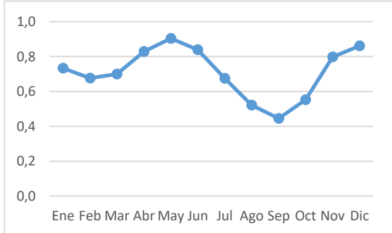
Caudal medio mensual (m³/s)
