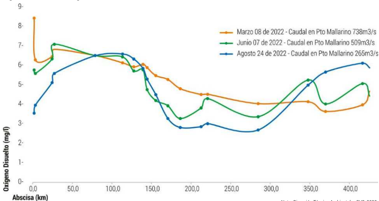
Figura 39. Perfil de oxígeno disuelto. Río Cauca, año 2022
