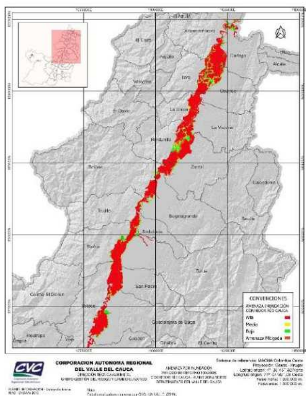
Figura 60. Zonificación de amenaza por inundación, corredor río Cauca
