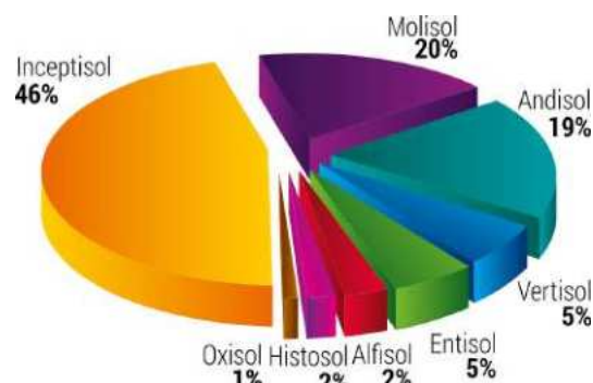
Figura 21. Ordenes de suelos en el departamento del Valle del Cauca
