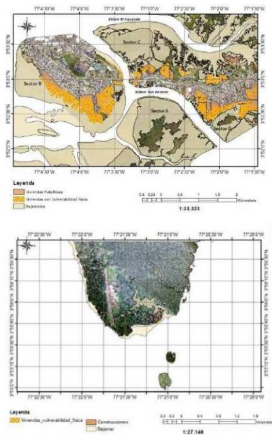
Figura 68. Definición zonas de mayor vulnerabilidad física en Buenaventura:
