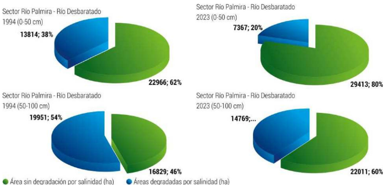
Figura 29. Comparación de los niveles de salinidad en el sector río Palmira-río Desbaratado de los años 2020-2023 frente a la línea base
