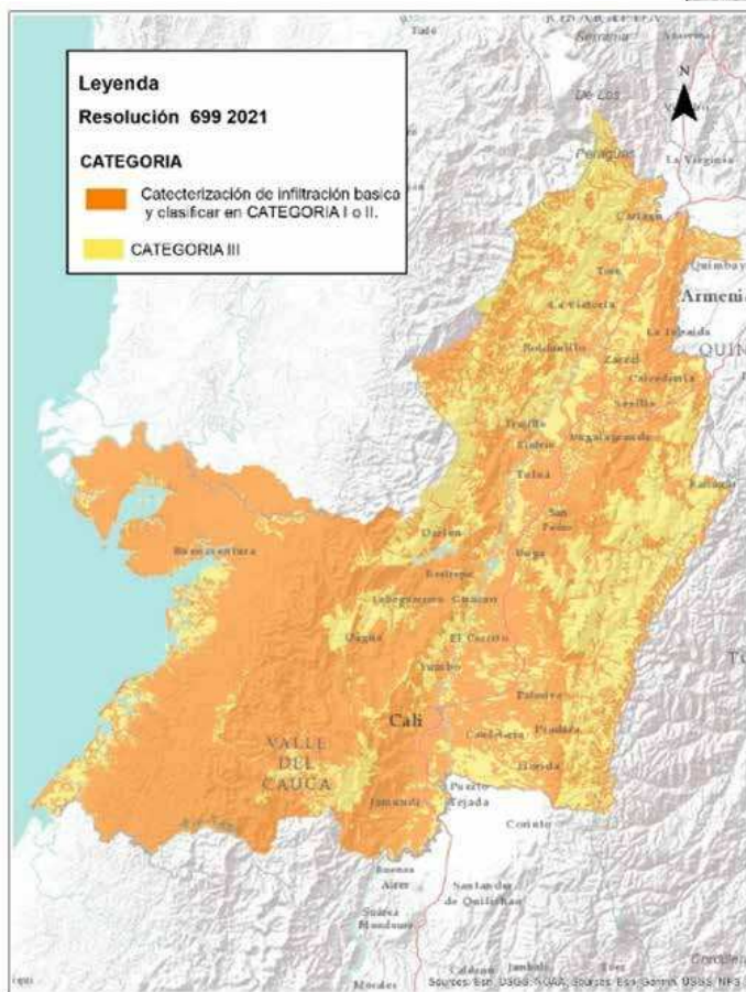
Figura 28. Mapa de categorías I y II en anaranjado y categoría III en amarillo claro, según Resolución 0699 de 2021
