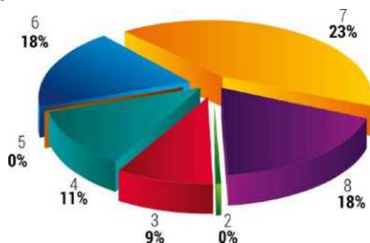
Figura 22. Clasificación agrológica de suelos en el departamento del Valle del Cauca
