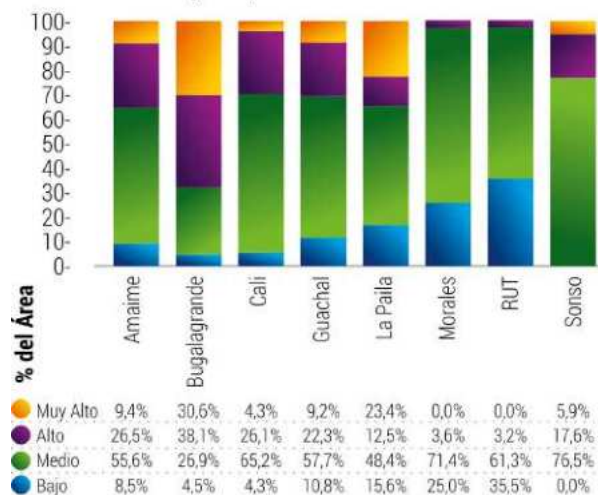
Figura 23. Distribución de categorías y contenidos de COS en las cuencas evaluadas
