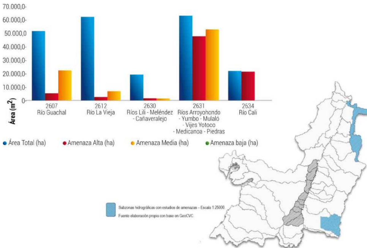
Figura 59. Amenaza categorizada por subzona hidrográfica para todos los eventos estudiados
