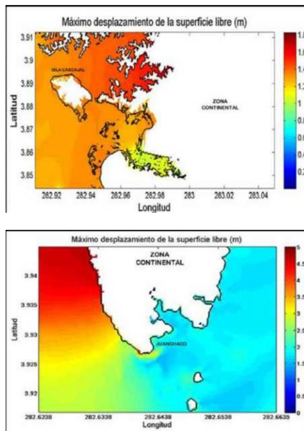
Figura 65. Propagación e inundación generada por el escenario sísmico E1. a) Casco Urbano de Buenaventura, b) Juanchaco.
