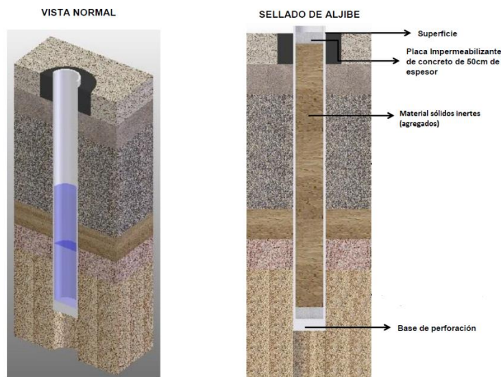
Esquema sellado de aljibe
