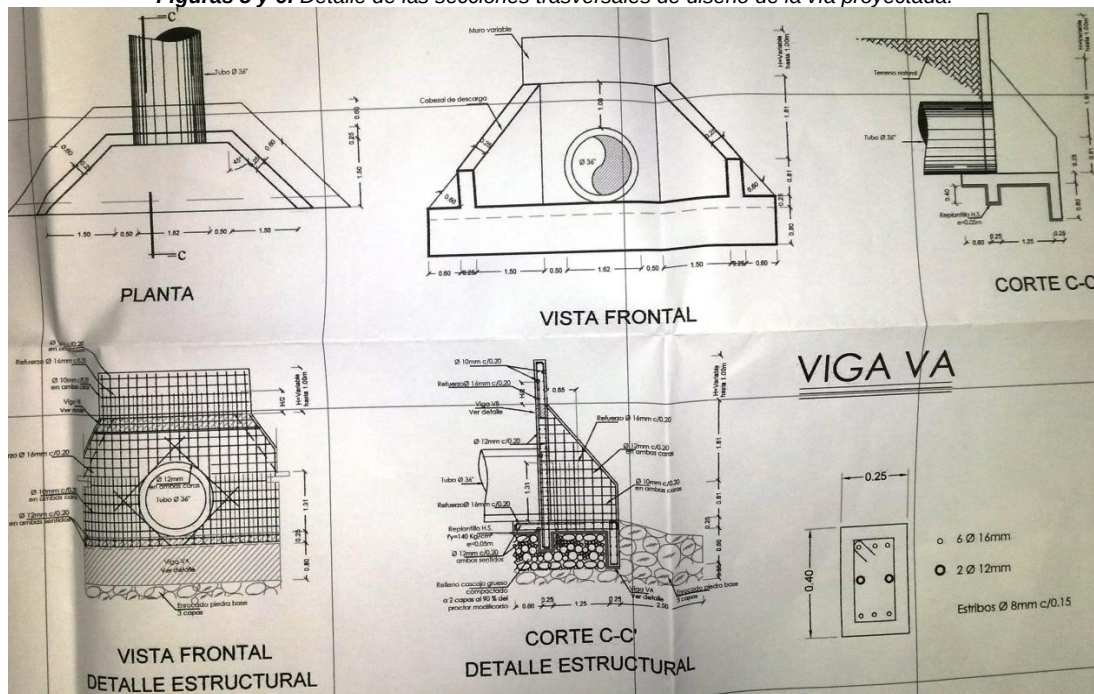
Figura 7: Detalle obra de alcantarilla tipo a implementar en el proyecto.
