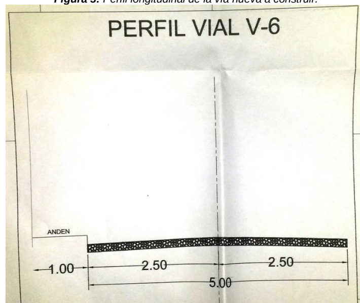
Figura 3: Detalle sección tipo de la vía.
