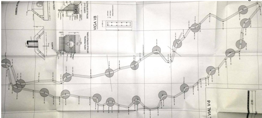
Figura 4: Detalle en planta de la vía proyectada y la localización de las obras complementarias.
